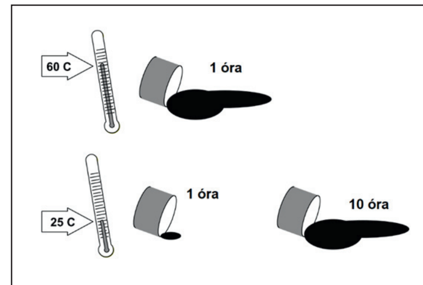
1. ábra. Ahogyan azt aszfalt viselkedik (Superpave Fundamentals Reference Manual 2010)
