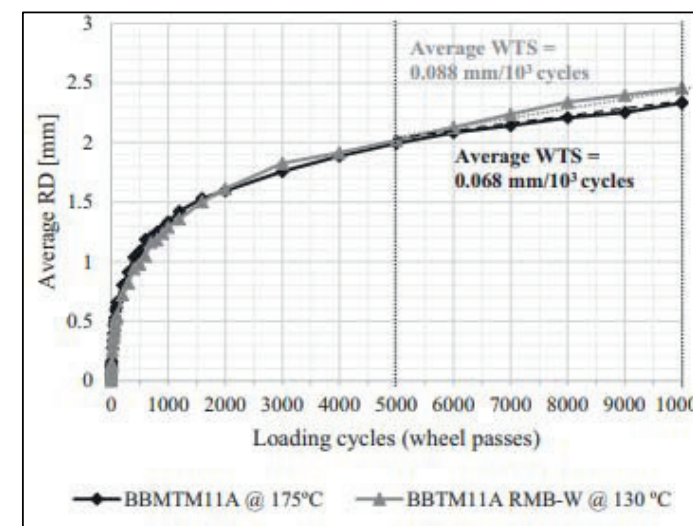
5. kép: Keréknyomképződési vizsgálat eredményei [18]
