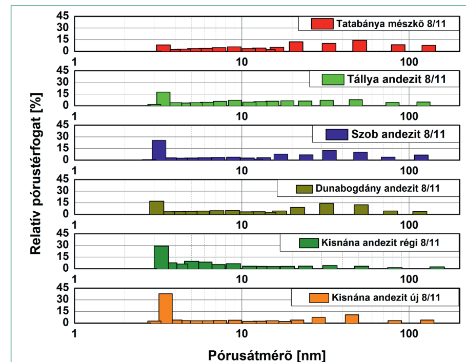
6. ábra. Különböző kőanyagok mikroporozitása (gázdeszorpciós módszer)
