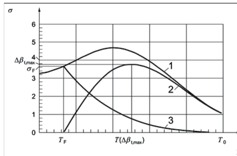
2. ábra – A vizsgálat során a próbatétel húzószilárdsága (1) és a próbatételben kialakuló termikus húzófeszültség (3) alakulása a hőmérséklet függvényében [MSZ EN 12697-46, 2012]
