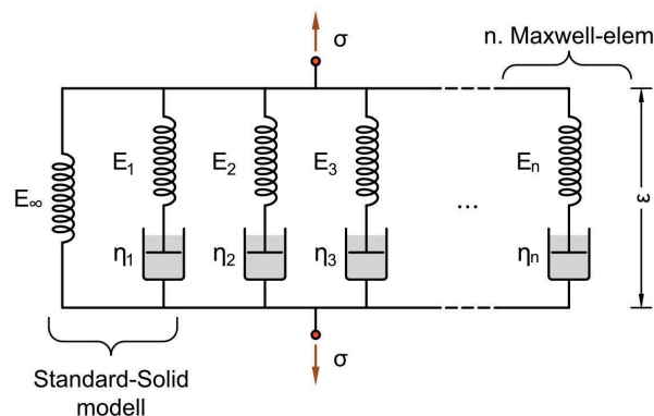
4. ábra. Az általánosított Maxwell-modell párhuzamosan kapcsolt Maxwell-elemből épül fel
