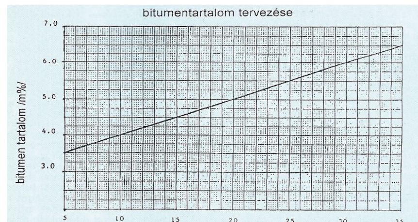
6. ábra: 0,075 mm-es szitán átesett anyag /m%/
