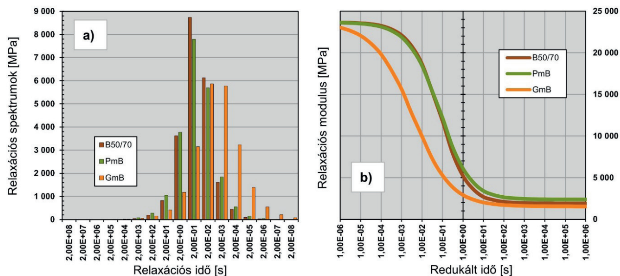
6. ábra. A három vizsgált aszfaltkeverék vonalas spektruma (a), és relaxáció függvénye (b)
