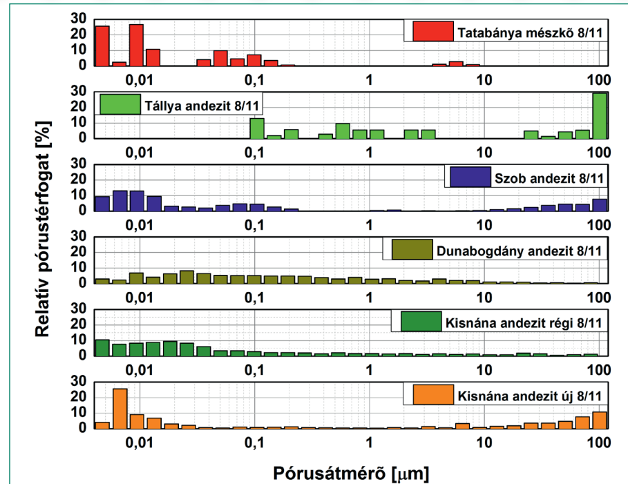
5. ábra. Különböző kőanyagok pórusméret-eloszlásai (higanyporozimetriás módszer)
