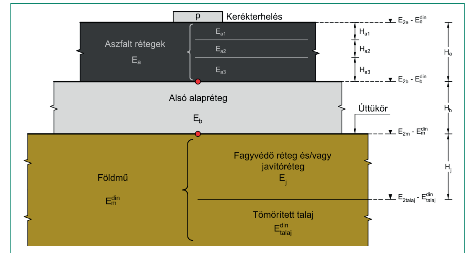
2. ábra – A Tóth-Primusz-féle analitikus eljárás szerkezeti modellje az ELZA felületén [Tóth, 2016a]
