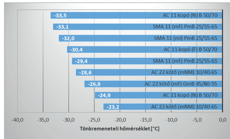
4. ábra – A vizsgált aszfaltkeverékek tönkremeneteli hőmérséklete
