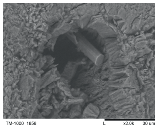
Szob andezit (N=2000 X)
