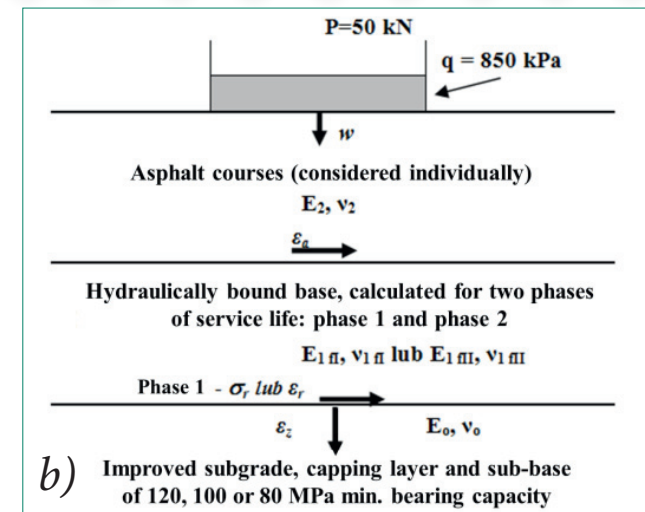
4. ábra. A számítások során alkalmazott modellek, a) rugalmas réteges féltér, b) félmerev burkolat felső szakaszainak modellje
