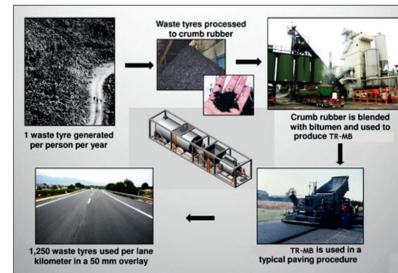
1.kép: Gumihulladékból gumibitumenes aszfalt keverék az USA-ban – gumihulladék hasznosításának sematikus ábrája [1]
