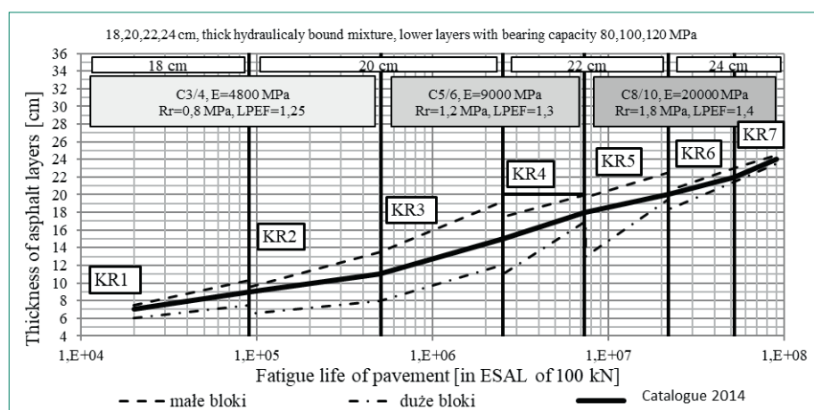
6. ábra: Félmerev burkolat fáradási élettartama hidraulikusan kötött alappal, az AASHTO 2004 fáradtsági kritérium alkalmazásával számolva
