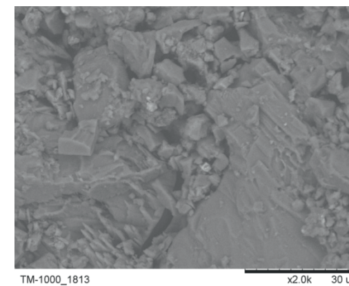
d) Dunabogdány andezit
