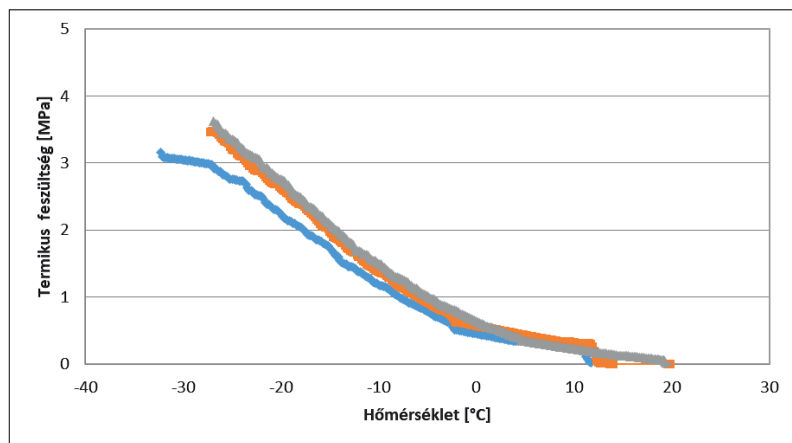
3. ábra – A termikus húzófeszültségek alakulása a gátolt alakváltozású aszfalt próbatestekben a TSRST vizsgálat során
