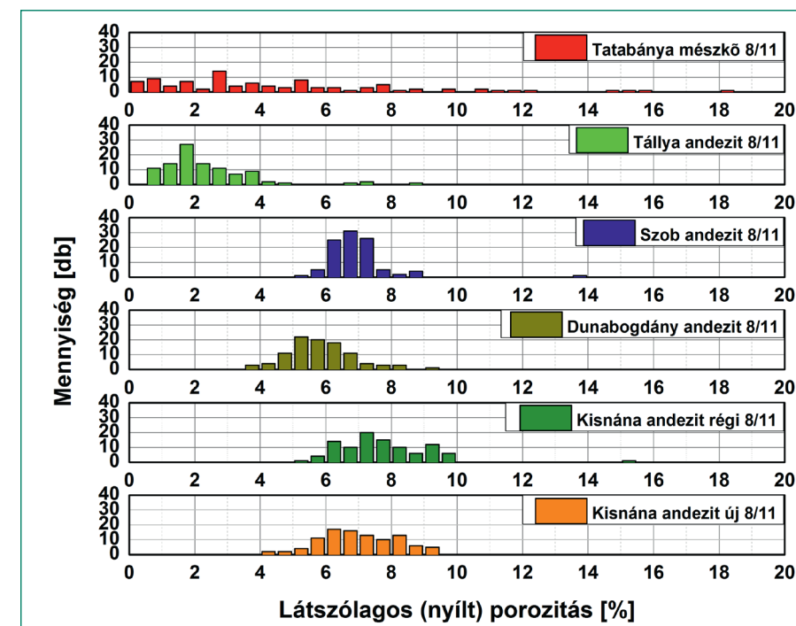
4. ábra. Különböző kőanyagok látszólagos (nyílt) porozitása
