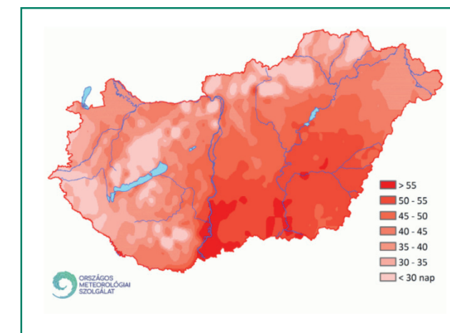
6a. és 6b. ábrák – A hazai forró napok száma 2019-ben illetve a hőhullámos napok száma az 1981–2016-es időszakban
