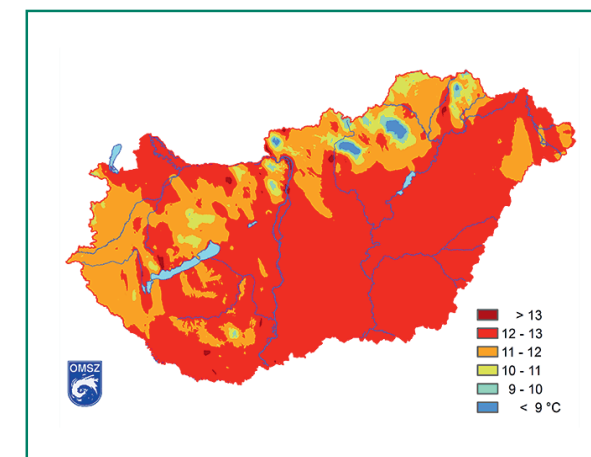
5a. és 5b. ábrák – Az évi középhőmérséklet területi eloszlása 2018. évben (5a. ábra) és 2019. évben (5b. ábra)
