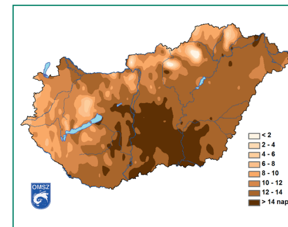
6a. és 6b. ábrák – A hazai forró napok száma 2019-ben illetve a hőhullámos napok száma az 1981–2016-es időszakban
