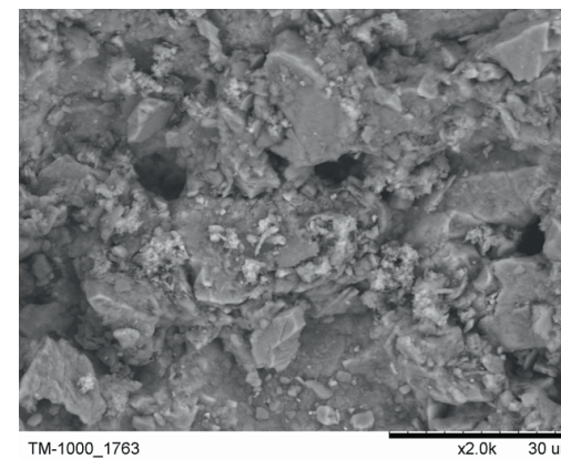
a) Tatabánya mészkő
