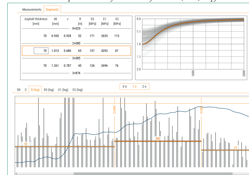
7. ábra - Mértékadó teherbírási paraméterek \sigma = 1 esetén
