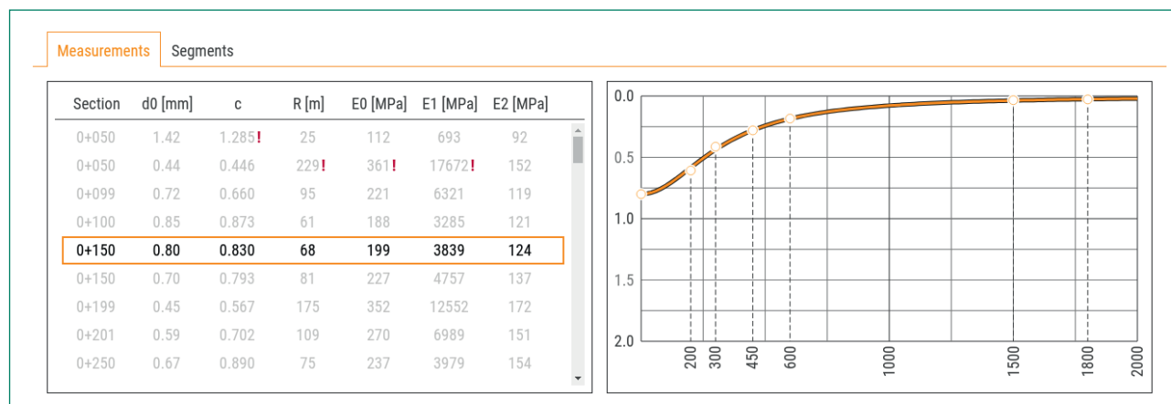
2. ábra - A kijelölt szelvényben kialakuló behajlási teknő és a számított teherbírási paraméterek
