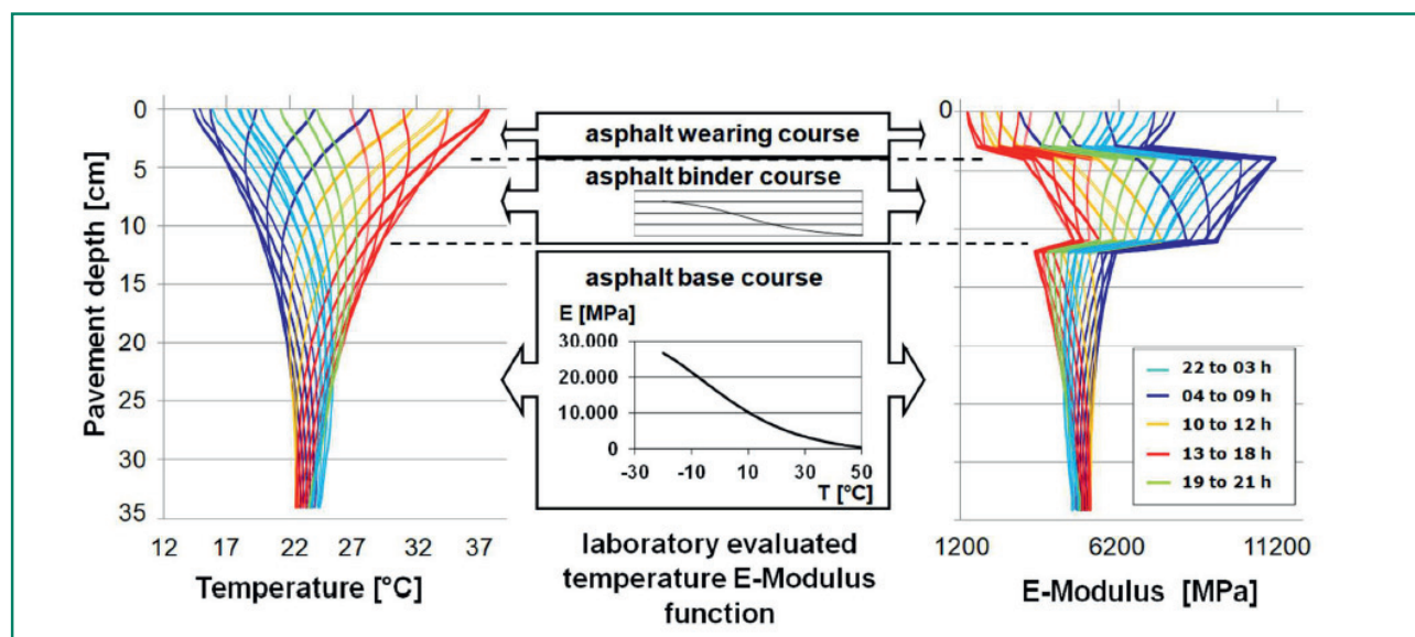
7. ábra - A pályaszerkezeti aszfaltrétegekben előforduló hőmérsékletek és az azoktól függő merevségi modulus ábrázolása a pályaszerkezet mélységében [Wistuba, 2018]
