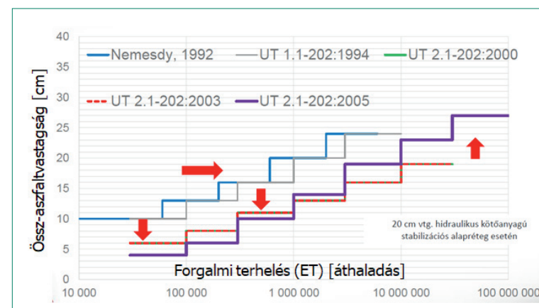
1. ábra – Az össz-aszfaltvastagságok alakulása a forgalmi terhelések függvényében a hazai előírások szerint [Tóth, 2016a]
