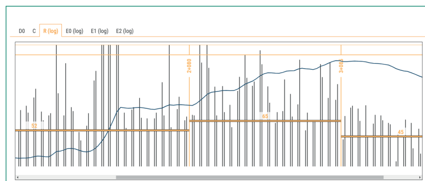
5. ábra - Homogén szakaszok a hossz-szelvényen
