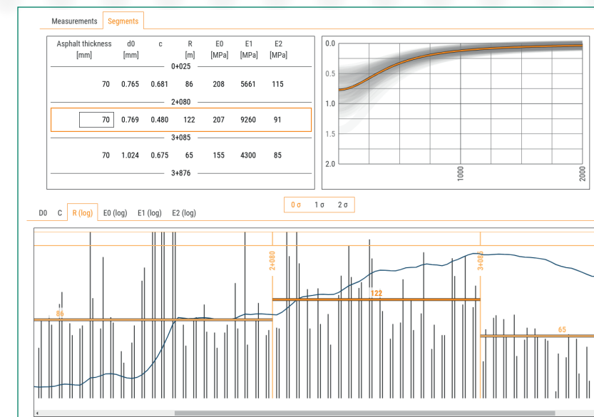
6. ábra - Teherbírási paraméterek a jellemző behajlási teknő ( \sigma = 0 ) alapján számítva
