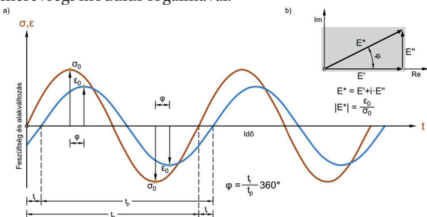
2. ábra. Az aszfaltanyag válasza zérus középpértékű, tiszta szinuszos lüktető gerjesztésre (a); a komplex rugalmassági modulus és összetevői a komplex síkon (b)
