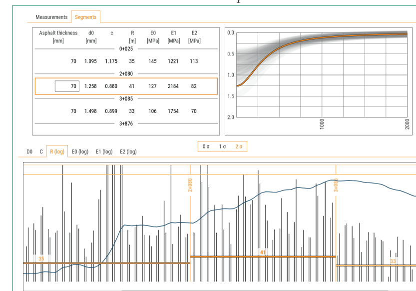
8. ábra - Mértékadó teherbírási paraméterek \sigma = 2 esetén
