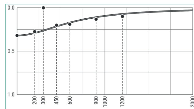
A 3. szenzor hibás mérése nem befolyásolja a behajlási teknő alakját ( D_0=0,32 mm, c=0,215 )
