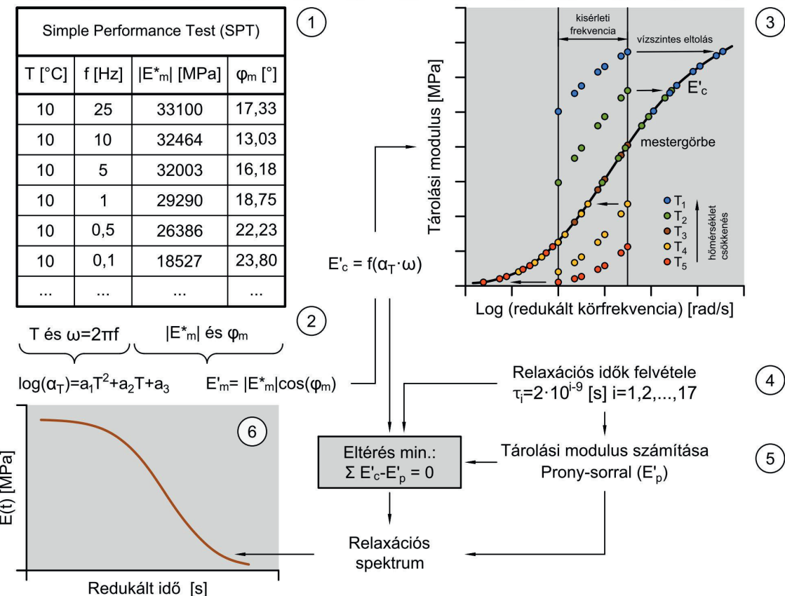
5. ábra. A relaxációs modulus meghatározásának folyamatábrája
