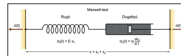
3. ábra. A Maxwell-teszt egy elastikus és egy viszkozus elem soros kapcsolásával jön létre
