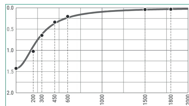
1. ábra - Fwd mérésre illesztett behajlási teknő ( D_0=1,42 mm, c=1,285 )
