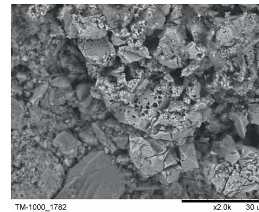
b) Tállya andezit
