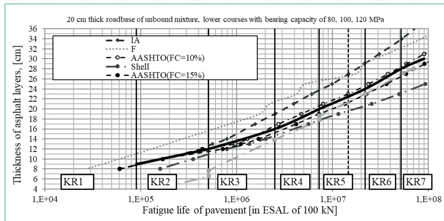
5. ábra: Kötőanyag nélküli alapú rugalmas burkolat (C90 / 3), 20 cm vastagságú fáradási élettartama, különböző fáradási kritériumok alkalmazásával számítva
