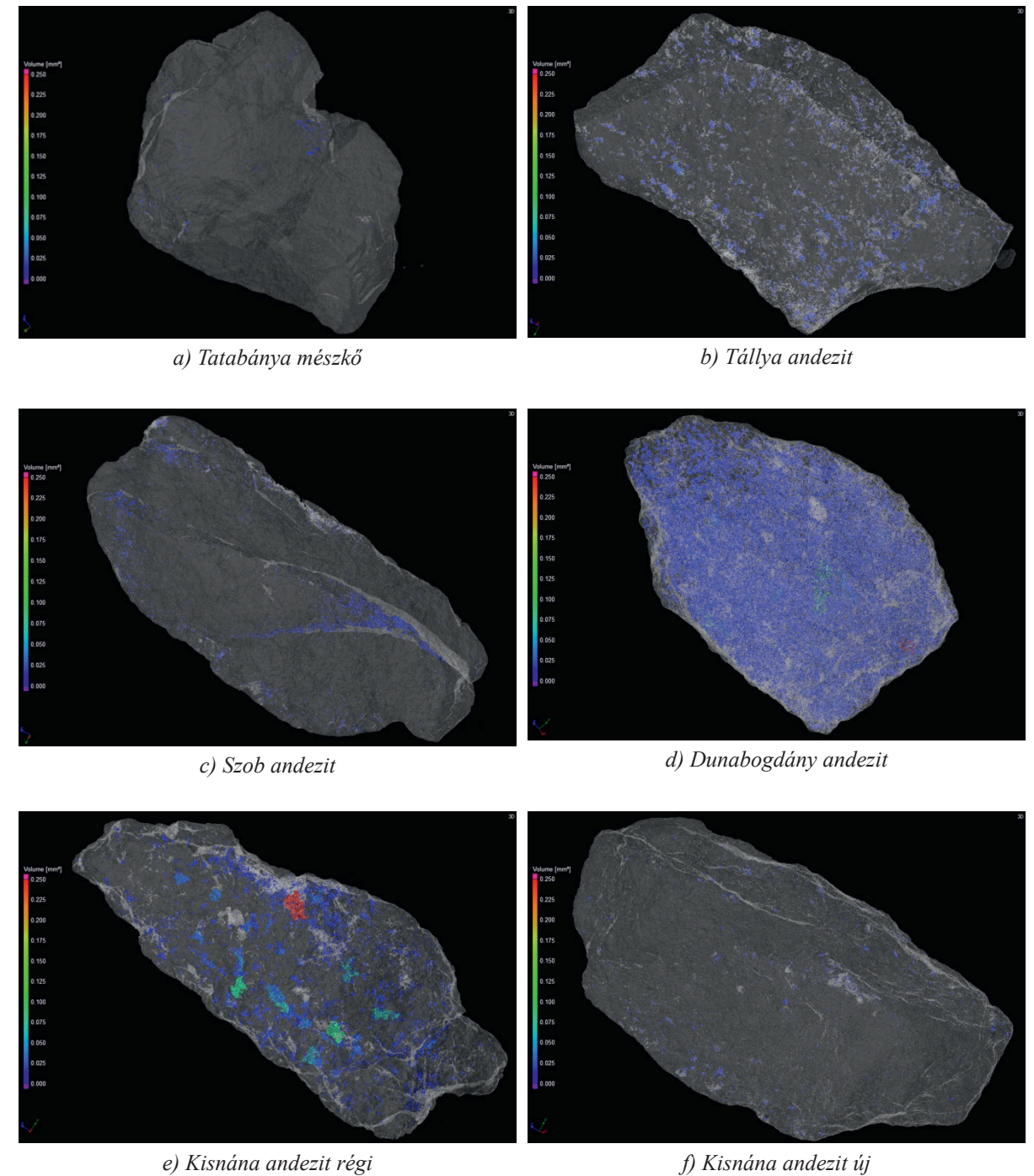
7. ábra. Kőanyagok zárt pórusainak térfogati eloszlása
