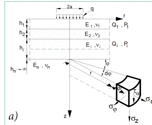
4. ábra. A számítások során alkalmazott modellek, a) rugalmas réteges féltér, b) félmerev burkolat felső szakaszainak modellje
