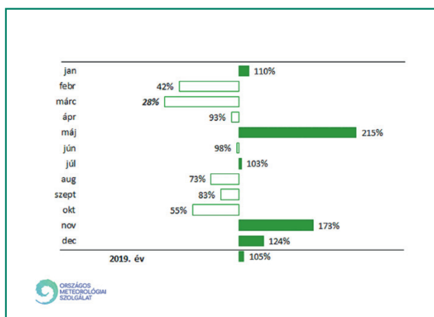
4a. és 4b. ábrák – A 2018. és 2019. évi havi csapadékösszegek változása az 1981-2010. évi normál (100%) százalékában
