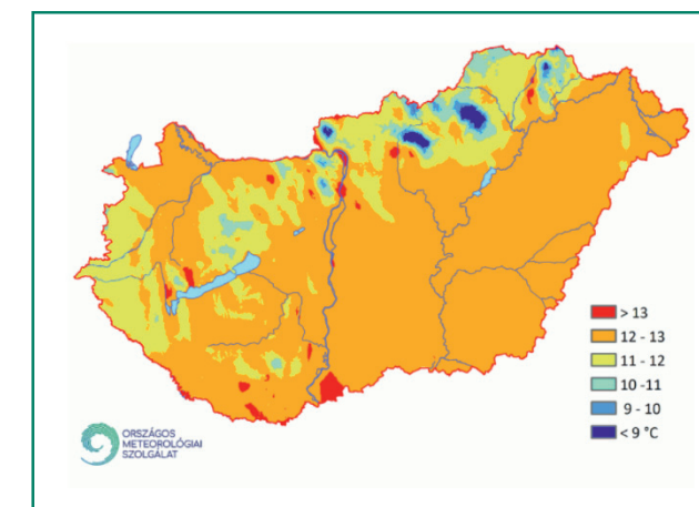
5a. és 5b. ábrák – Az évi középhőmérséklet területi eloszlása 2018. évben (5a. ábra) és 2019. évben (5b. ábra)
