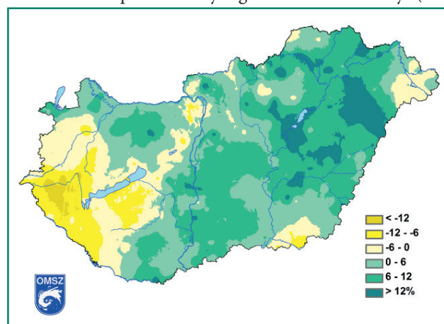
3a. és 3b. ábrák – A 2019. évi csapadékösszegek illetve az 1961 és 2016 közötti éves csapadékösszegek változása országos eloszlásban
