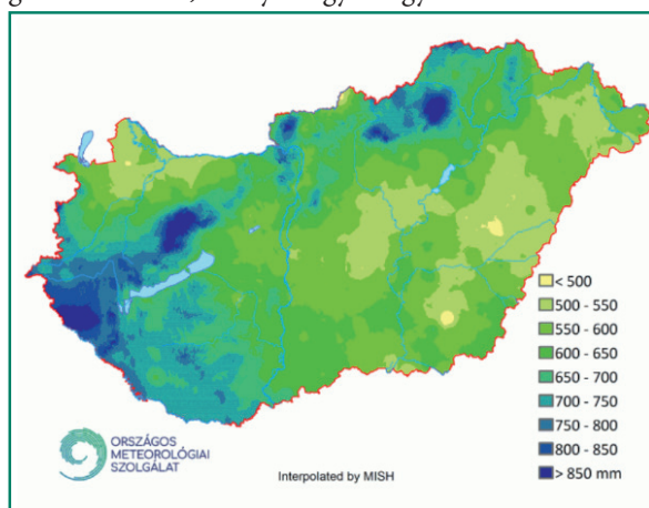
3a. és 3b. ábrák – A 2019. évi csapadékösszegek illetve az 1961 és 2016 közötti éves csapadékösszegek változása országos eloszlásban
