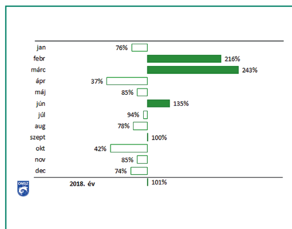
4a. és 4b. ábrák – A 2018. és 2019. évi havi csapadékösszegek változása az 1981-2010. évi normál (100%) százalékában
