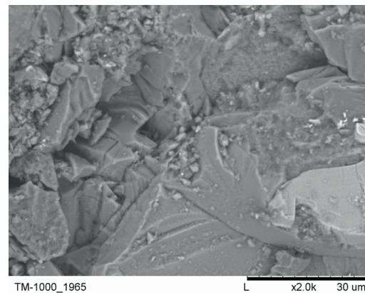
f) Kisnána andezit - új
