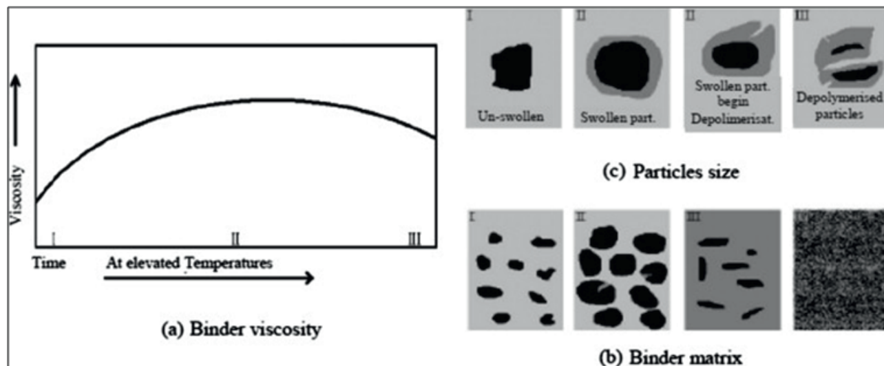
2. kép: Kötőanyag viszkozitás alakulása a gumi őrlémény és bitumen érintkezése esetén, gumi részecskék duzzadási és oldódási folyamata [10]
