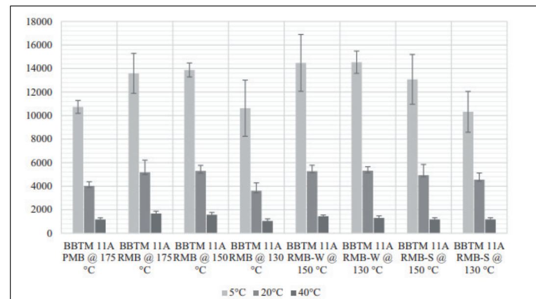
4. kép: A BBTM 11A keverékek merevségi (MPa) eredményei különböző vizsgálati hőfokon. [18]
